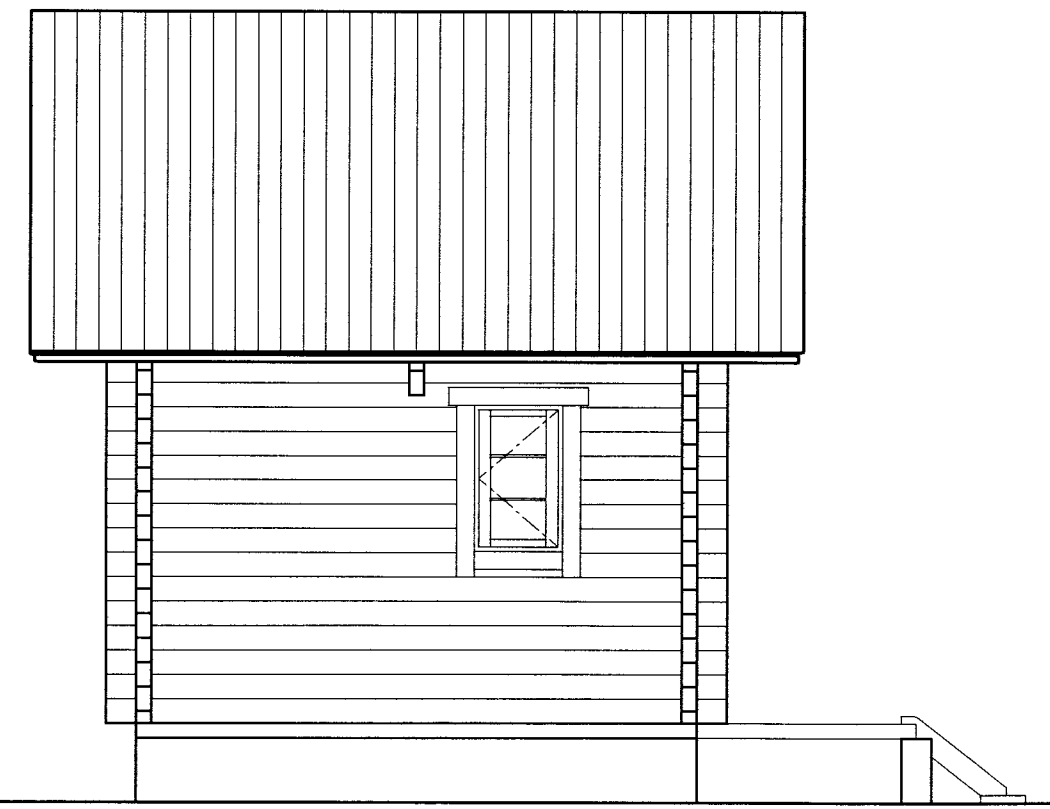
立面図 S=1/50
