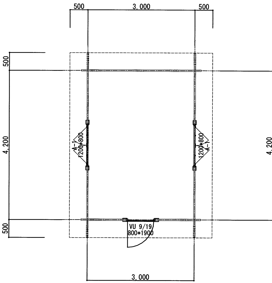
平面图 S=1/50
