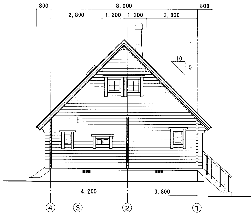
北側立面図 1:100
