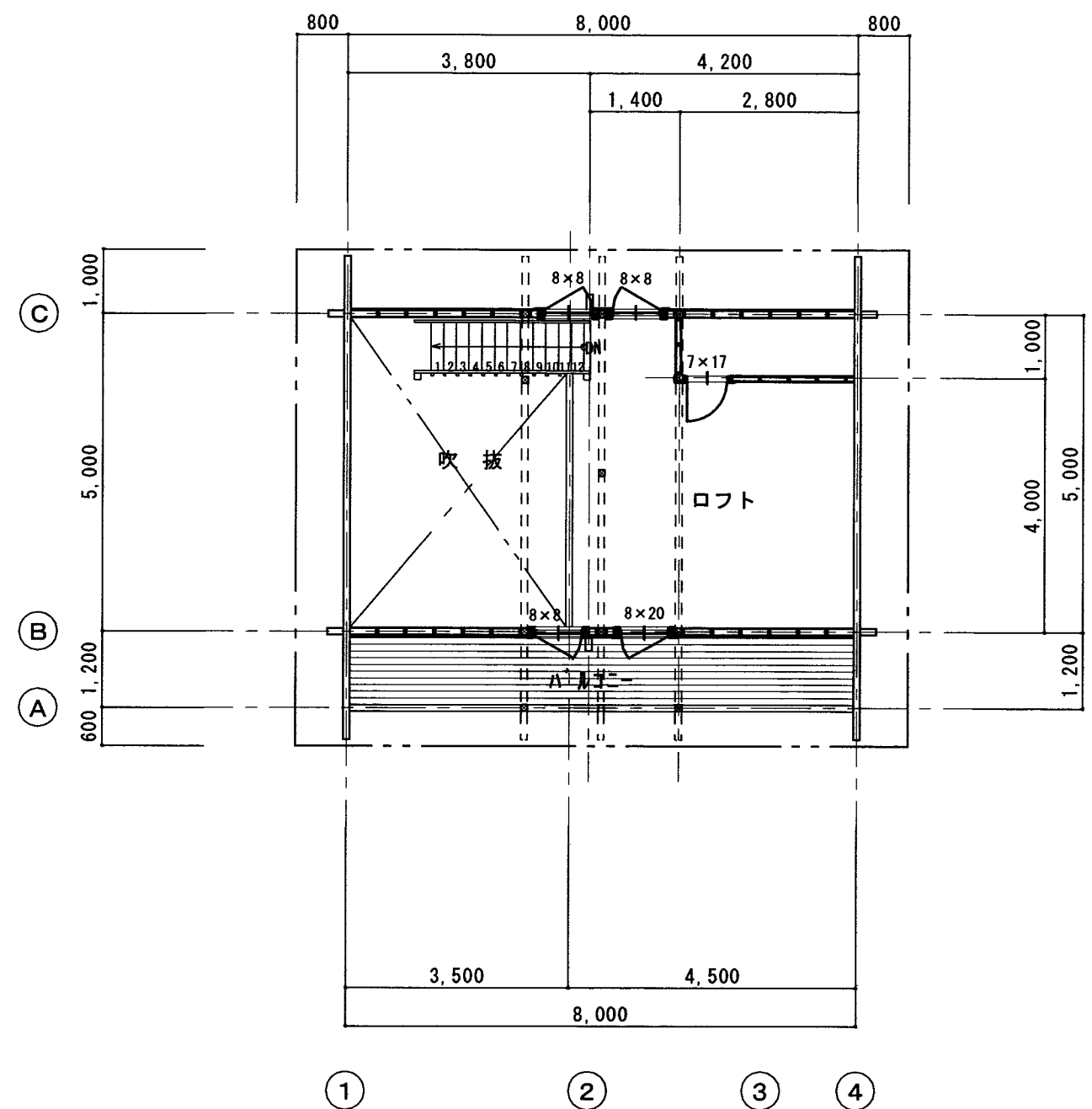
2階平面図 1:100
