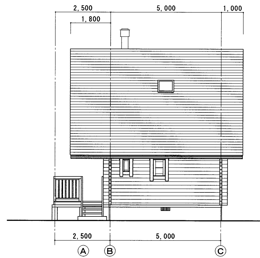
西側立面図 1:100
