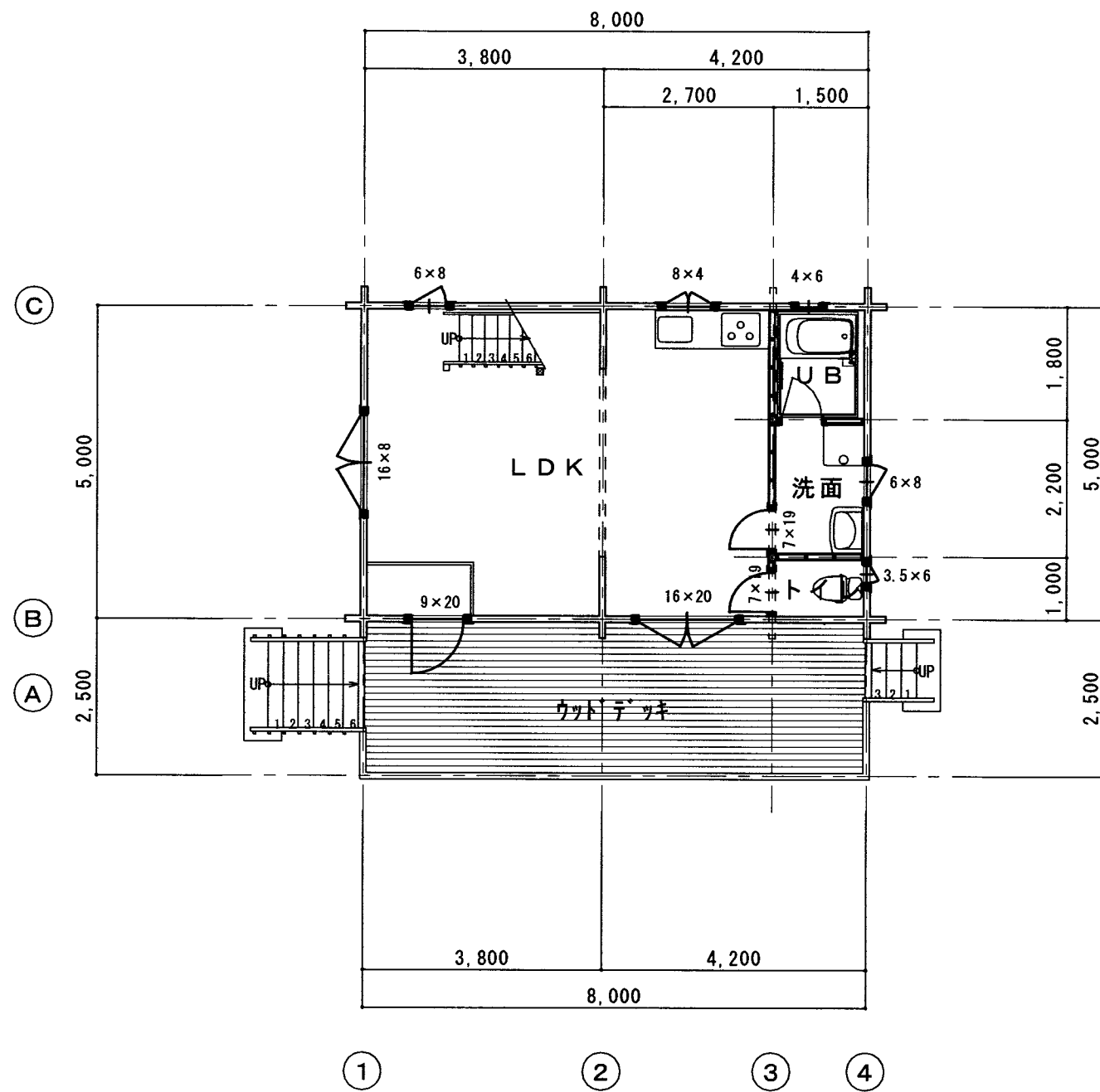
1階平面図 1:100
