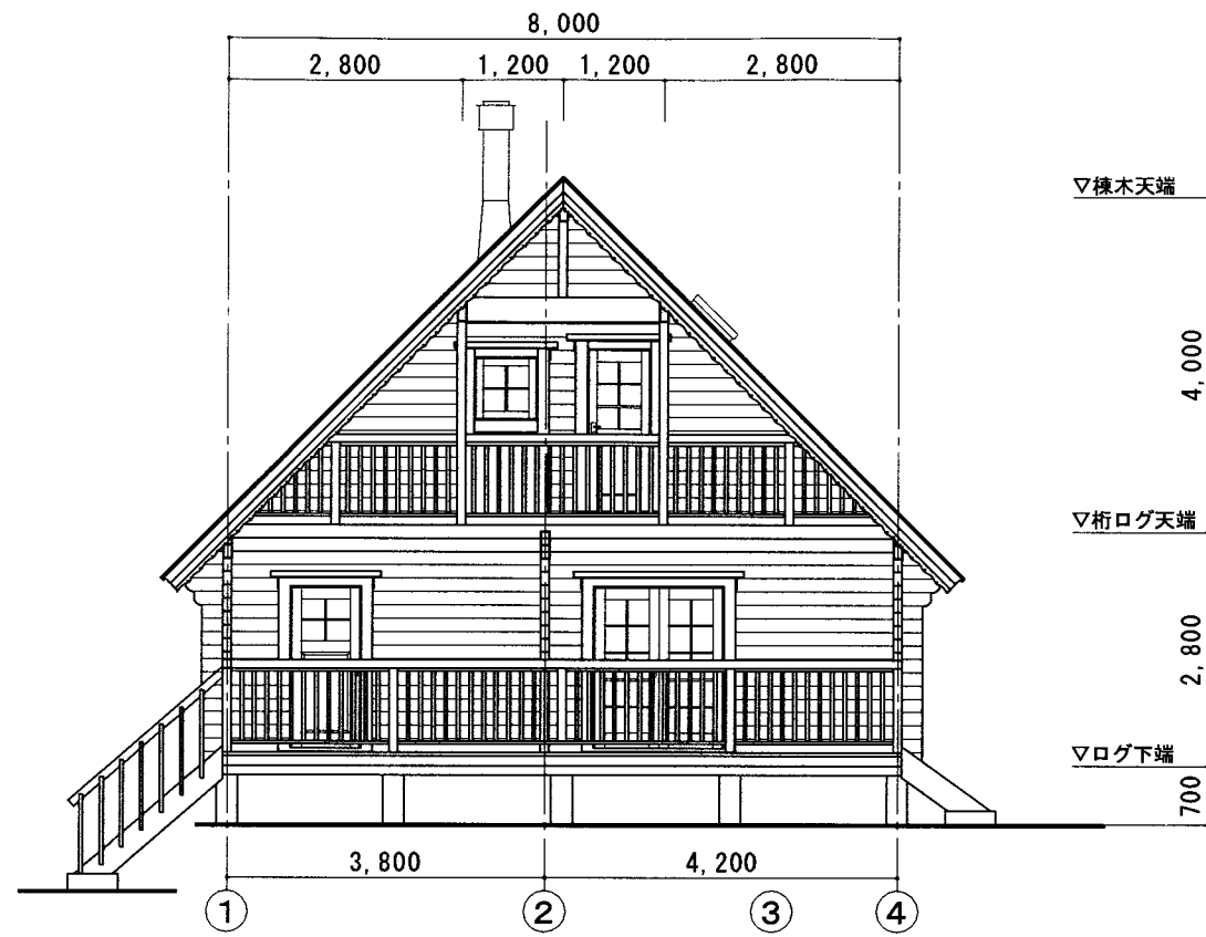
南側立面図 1:100
