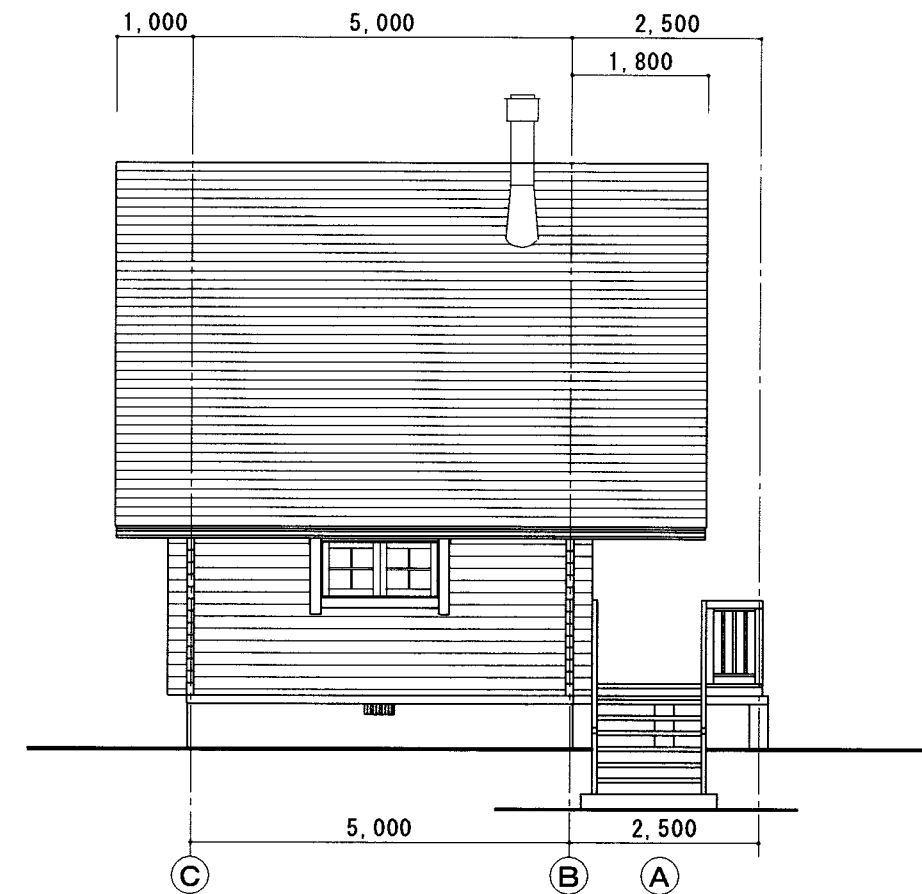
東側立面図 1:100
